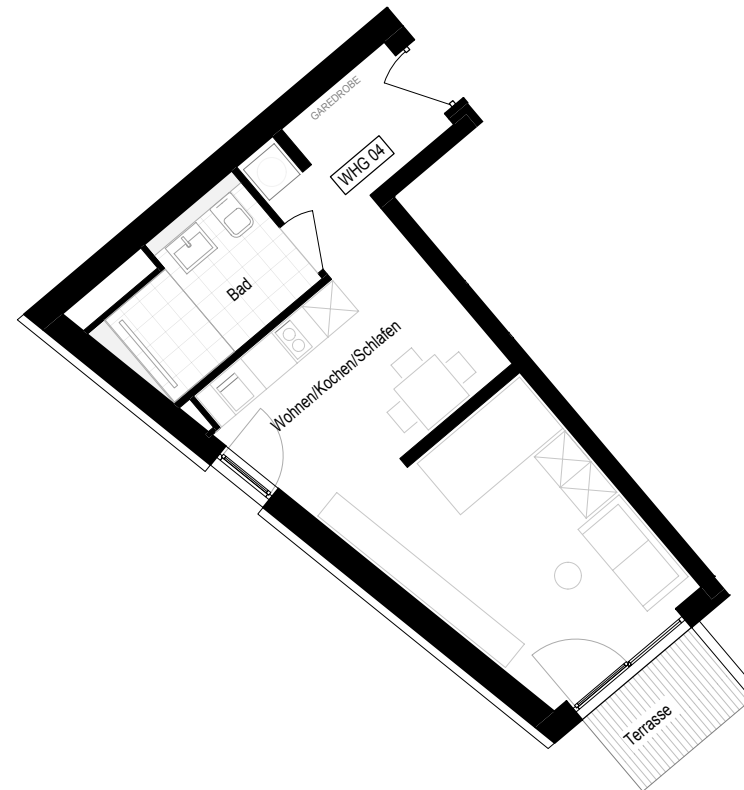
Neubau Erdgeschoss Einzimmer-Apartment WHG 04
