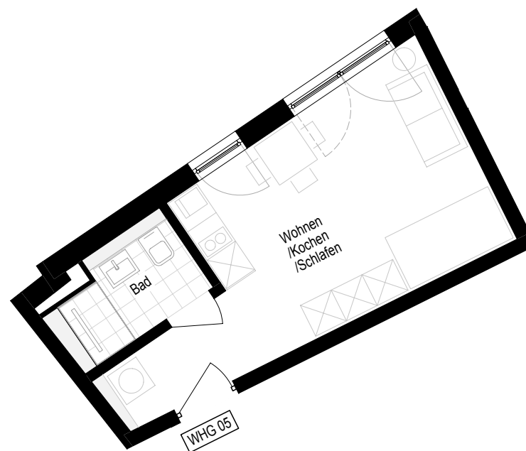
Neubau 1. Obergeschoss Einzimmer-Apartment WHG 05
