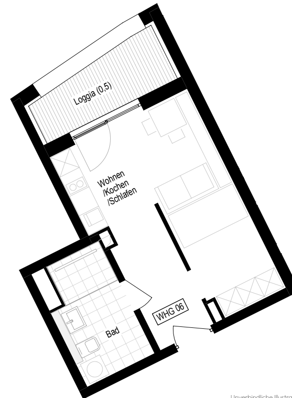
Neubau 1. Obergeschoss Einzimmer-Apartment WHG 06
