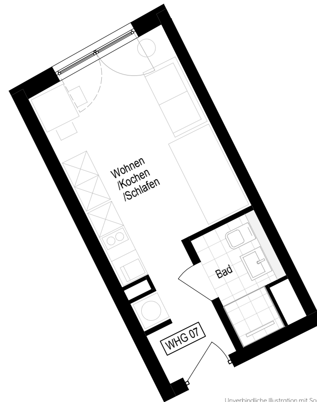
Neubau 1. Obergeschoss Einzimmer-Apartment WHG 07
