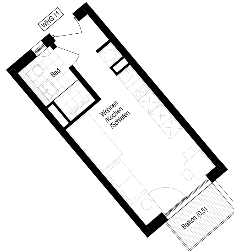
Neubau 1. Obergeschoss Einzimmer-Apartment WHG 11
