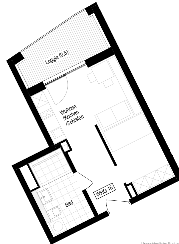
Neubau 2. Obergeschoss Einzimmer-Apartment WHG 16
