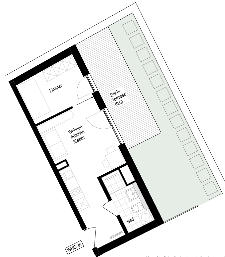
Neubau 3. Obergeschoss Zweizimmer Wohnung WHG 26
